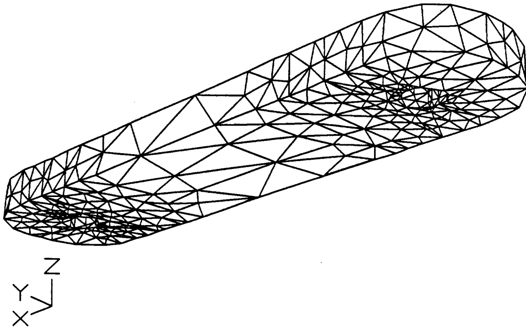
Fig. 2 Torque Arm Mesh
