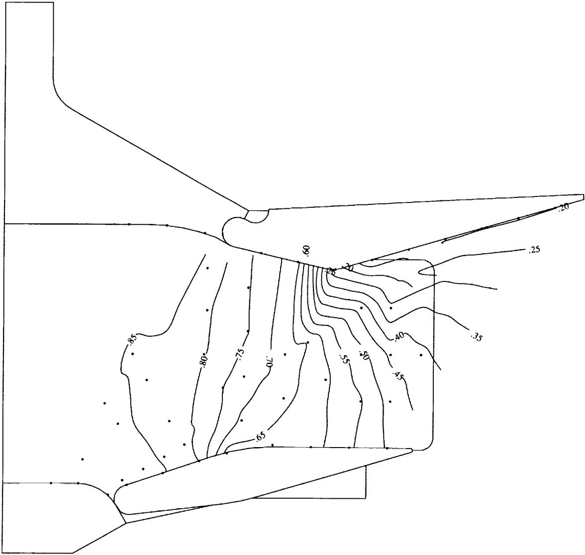
(d) Max 0° configuration. NPR = 5.0.
