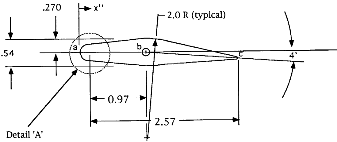
(d) Lower rotating flap.
