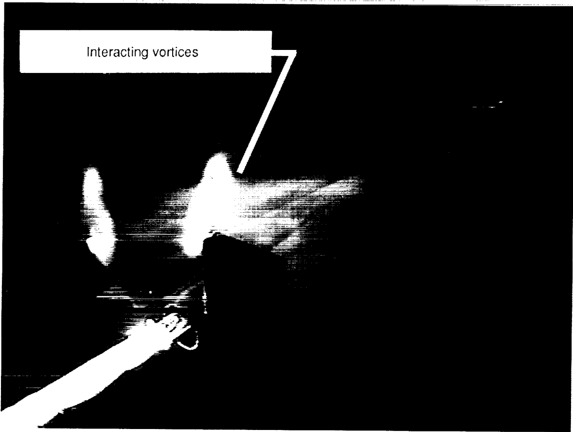
(d) Vortex-vortex and vortex-tail interactions aft of tails.
