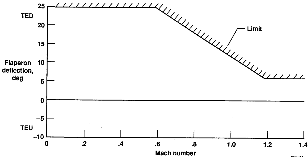
(b) Flaperon.
