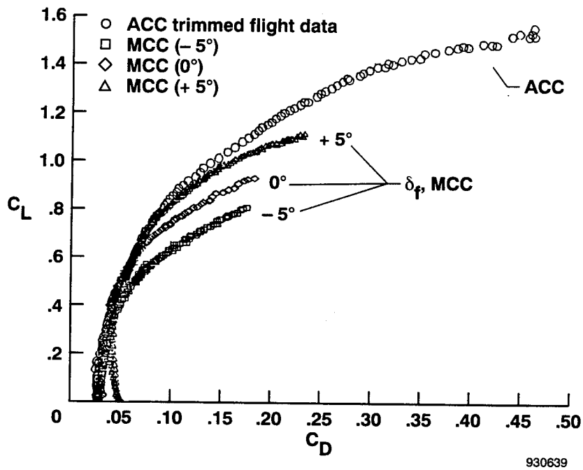
(b) Drag polar.
