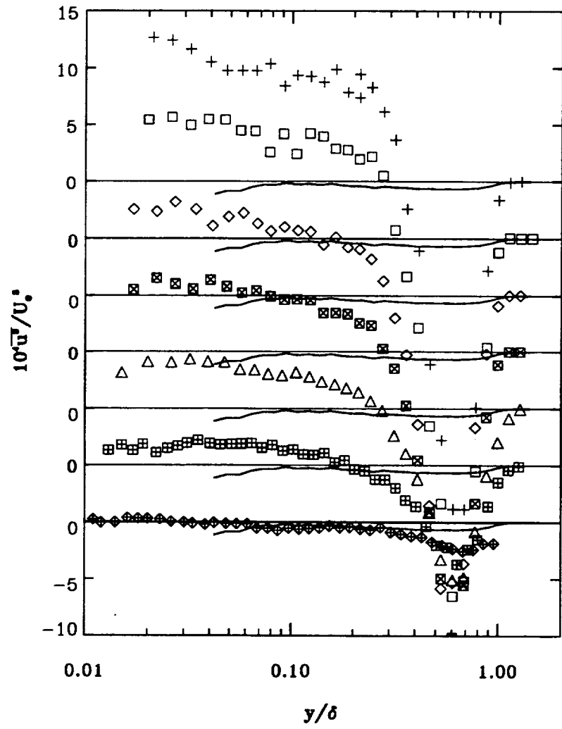
Figure 12. Concluded. (d) \overline{u^3} .
