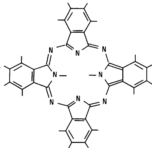
FIGURE 4.—Metal-free Pc ( \text{H}_2\text{Pc} ).
