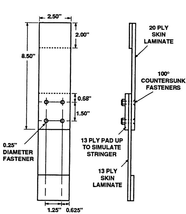
LONGITUDINAL SKIN SPLICE SPECIMEN
