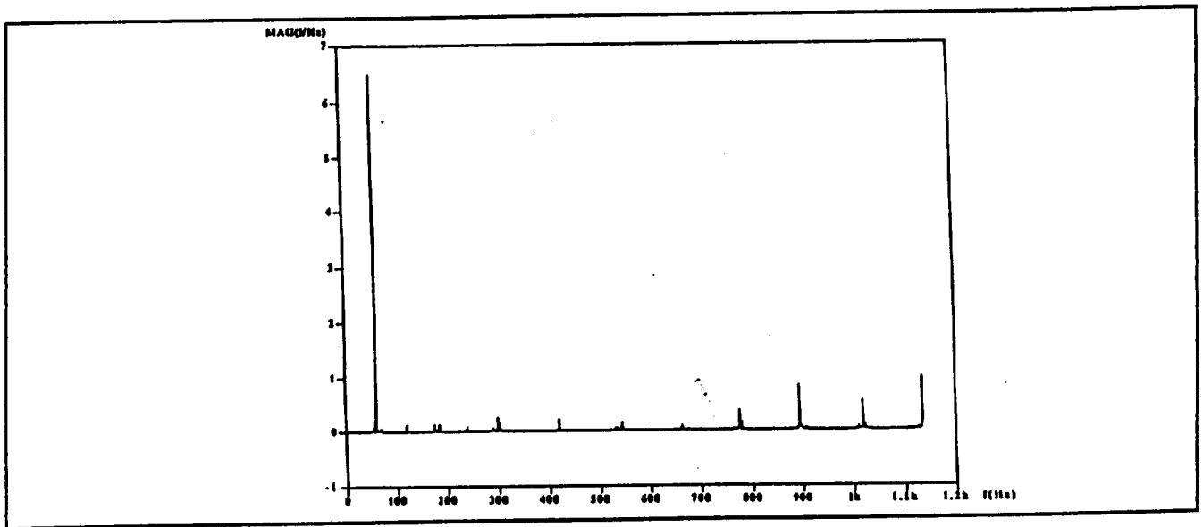
Figure 16. FFT Analysis of IM Current of Fig 16.
