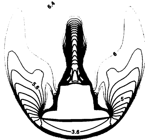
f) Fuselage cross-section transition ( x/L=0.54 ).
