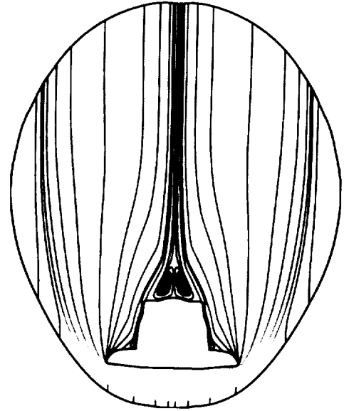
f) Fuselage cross-section transition ( x/L=0.54 ).
