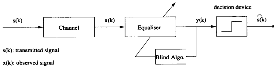
FIG. 1.1. Blind Equalisation
