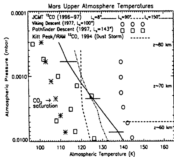
Fig. 3. Temperatures in the Mars mesospheres.
