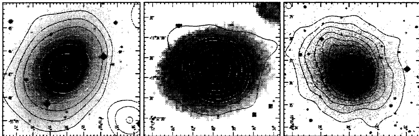
NGC 1553
