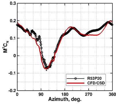
(d) M^2 C_n, r/R = 0.865
