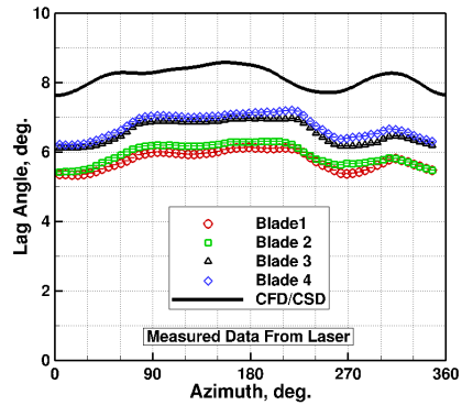
(h) Lag: Laser Data
