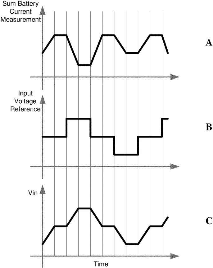
MPPT Mode FIG. 7
