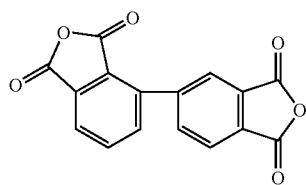
(6) a-BPDA
