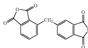
(14) a-MDPA
