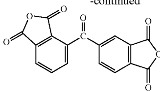
(10) a-BTDA
