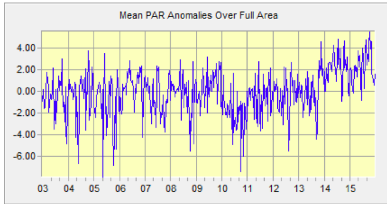
Figure 9. Mean PAR anomaly from 2003-2015. Y-axis values are in Einstein m^{-2} d^{-1} .
