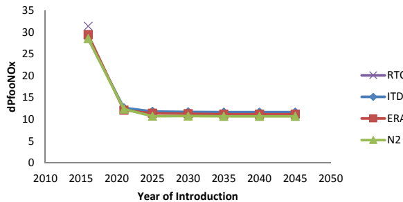
SSA - Conventional - dPfooNOx
