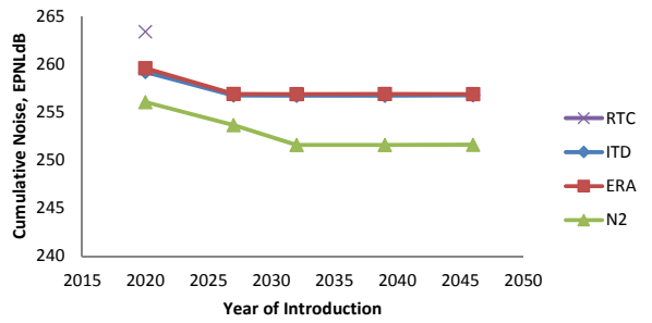
STA - UC1 - Cumulative Noise
