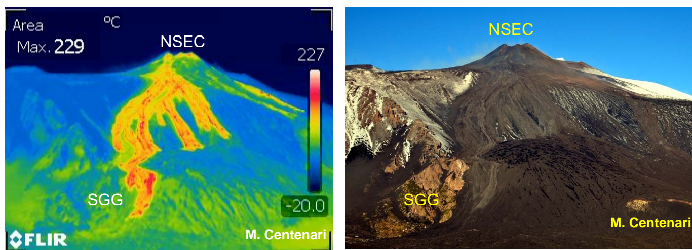
Fig. 2. Immagine termica e visibile ripresa da M. Zoccolaro alle ore 08:30 GMT del 17/12/13 che mostra le colate laviche in raffreddamento sviluppatasi lungo la parete occidentale della Valle del Bove. SGG= Serra Giannicola Grande; NSEC=nuovo cono del Cratere di Sud-Est.
