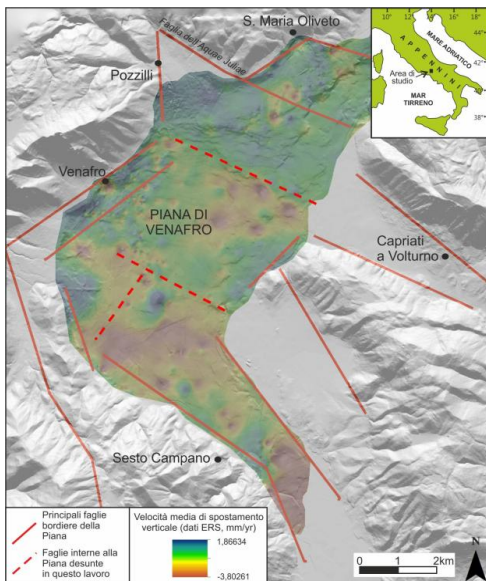
Fig. 1 □ DEM (scala 1:5000) con schema tettonico semplificato e distribuzione delle velocità medie degli spostamenti verticali
