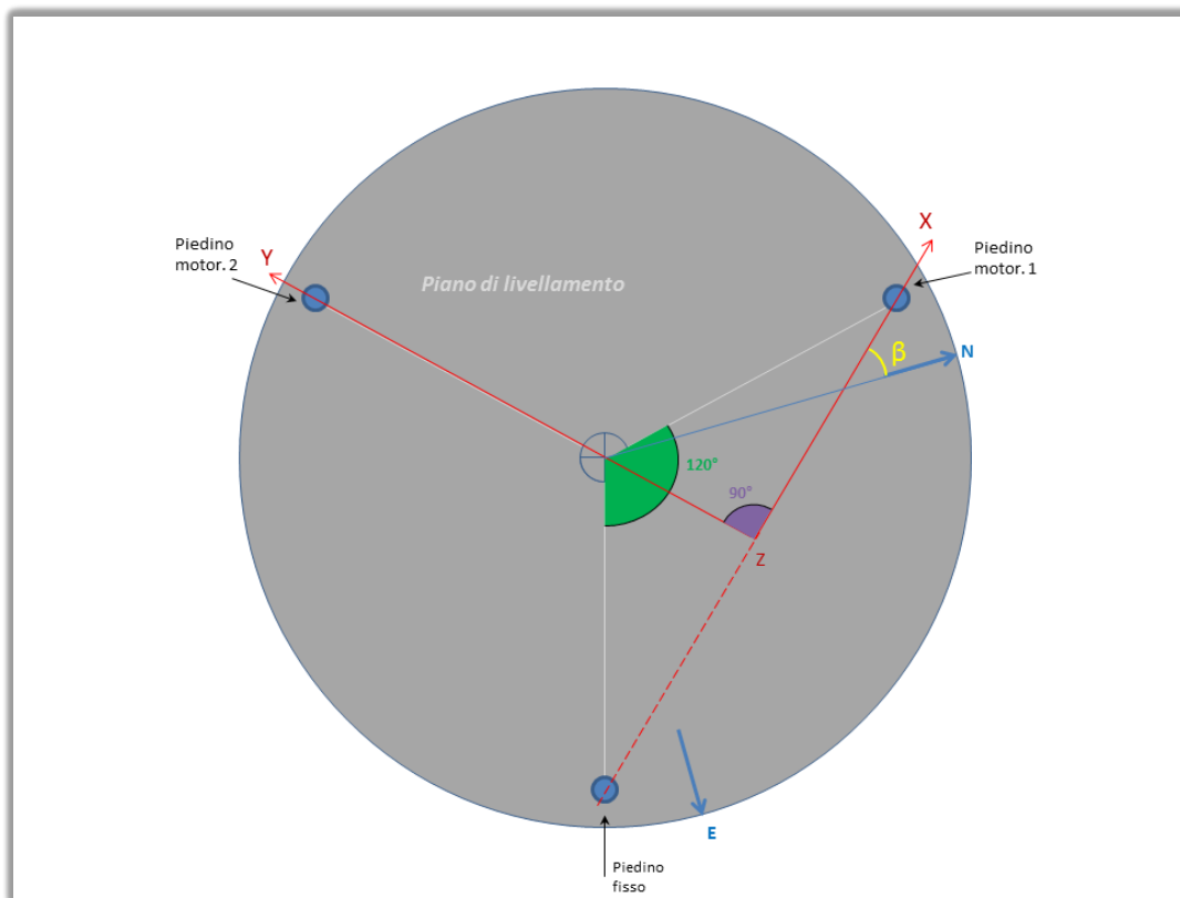
Figura 2. Geometria della base del Nanometrics Trillium 40s. Intersezione assi X,Y con gli assi dei piedini. Angolo \beta tra asse N-S e asse X.
