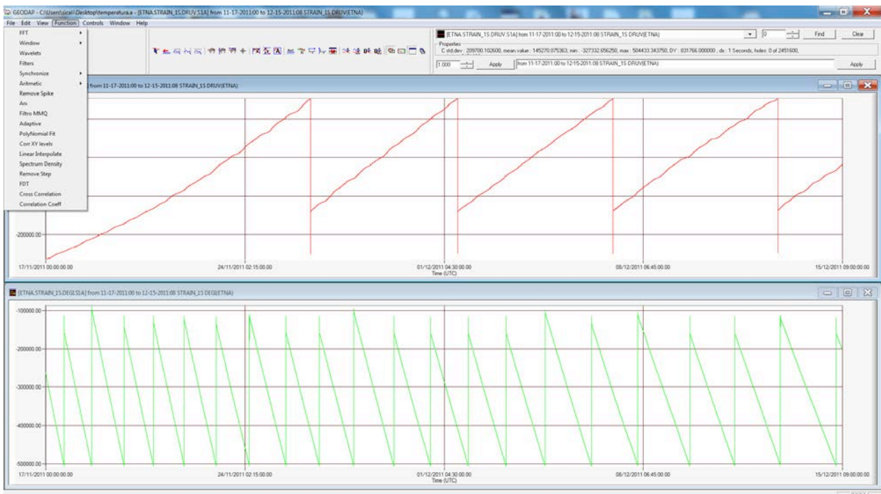
Figura 11. Schermata del software Geodap. I bruschi e marcati offset che caratterizzano il segnale sono relativi all'apertura della valvola che consente il riequilibrio dello strain cumulato.
