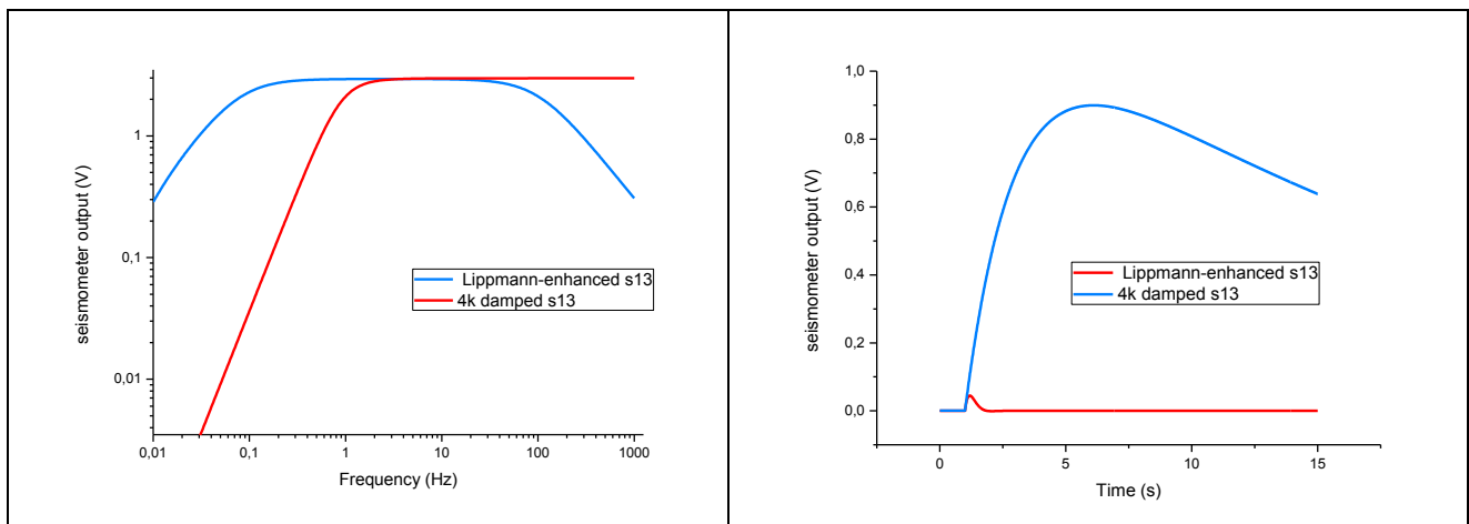
Figura 12. Risposta in frequenza ed al gradino dell'estensore di banda di tipo Lippmann illustrato in Figura 11. A sinistra notiamo che il taglio alle basse frequenze che passa da 1 a 0.1 Hz. Questo si traduce in una notevole risposta al gradino (a destra), il cui contenuto in bassa frequenza viene esaltato dall'aumento della estensione di banda. In queste simulazioni è stata ignorata l'induttanza della bobina di pick-up.
