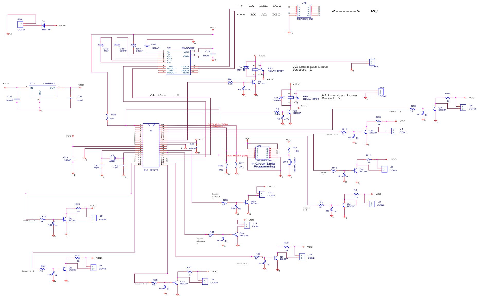
Figura 6. Schema elettrico del circuito.
