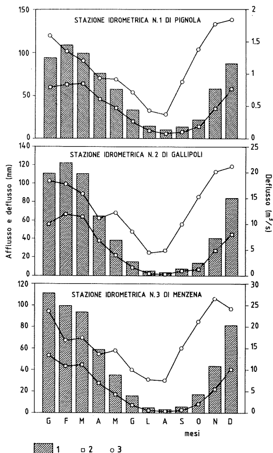
Fig. 2 - Afflusso-deflusso alle stazioni idrometriche. (1) deflusso m^3/s ; (2) deflusso mm; (3) afflusso mm.
