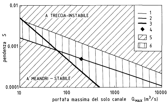
Fig. 12 - Caratteri idrogeomorfici e andamento fluviale: confronto tra 3 relazioni. (1) relazione di LEOPOLD & WOLMAN (1957), (2) relazione di BEGIN (1981), (3) relazione di BROOKES (AA.VV.; 1983); (4) Basento a Menzena, (5) le tre relazioni sono concordi, (6) solo due relazioni sono concordi.
