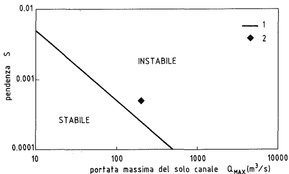
Fig. 9 - Caratteri idrogeomorfici e andamento fluviale: relazione di KELLER & BROOKES (AA.VV., 1983). (1) relazione di KELLER & BROOKES, (2) Basento a Menzena.
