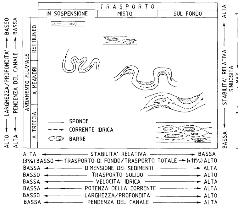
Fig. 8 - Andamenti fluviali, stabilità relativa e caratteristiche idrogeomorfiche. Da SCHUMM, 1981; modificata.
