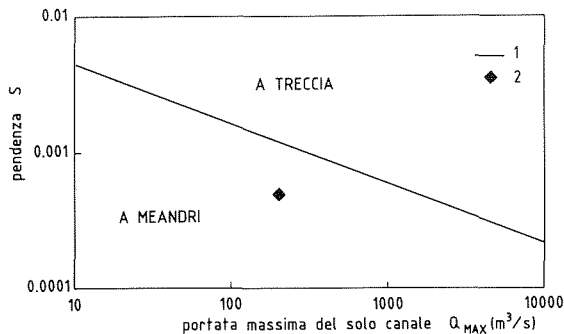
Fig. 10 - Caratteri idrogeomorfici e andamento fluviale: relazione di LEOPOLD & WOLMAN (1957). (1) relazione di LEOPOLD & WOLMAN; (2) Basento a Menzena.
