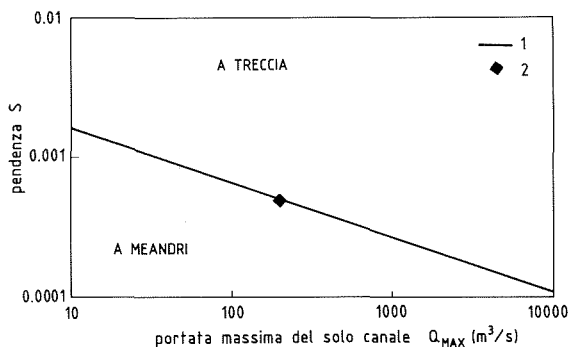
Fig. 11 - Caratteri idrogeomorfici e andamento fluviale: relazione di BEGIN (1981). (1) relazione di BEGIN; (2) Basento a Menzena.
