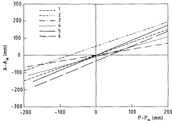
Fig. 17 - Variazioni nel tempo della relazione tra gli afflussi e le perdite. Rette di regressione relative alle differenze, calcolate anno per anno, A - A_m e P - P_m , relative alla stazione idrometrica: Pignola, (1) 1926-1971, (2) 1961-1971; Gallipoli (3) 1927-1971, (4) 1961-1971; Menzena, (5) 1939-1971, (6) 1961-1971.
