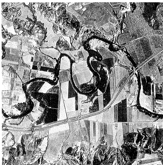
Fig. 5 - Modificazioni dell'alveo del F. Basento in località Mass. Nobile (A) e a monte della confluenza del Fosso La Canala (B). (Aerofotografie dell'Archivio Topografico dell'I.G.M.I., Concessione S.M.A. n. 329 del 23/5/1970 e n. 477 del 13/5/1992. La cartografia di tav. 1 deriva dai tipi dell'I.G.M.I. con autorizzazione n. 3612 del 30/4/1992).
