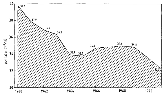
Fig. 18 - Differenza tra il deflusso alle stazioni idrometriche di Menzena e di Gallipoli. Calcolata tale differenza anno per anno e la media progressiva al crescere degli anni di osservazione, è rappresentato l'andamento di tale media negli ultimi dieci anni disponibili.
