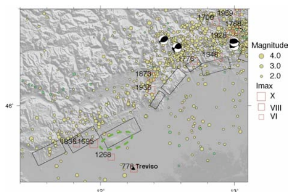
Figura 1. Mappa dell'area in esame: la linea tratteggiata in verde indica il Montello. I cerchietti indicano gli epicentri degli ultimi 30 anni, con sorgente superficiale < 30\text{km} (gialli), e più profonda (verdi). Sono riportati gli eventi storici, i momenti tensore [Pondrelli et al., 2002] e le sorgenti sismogenetiche.
