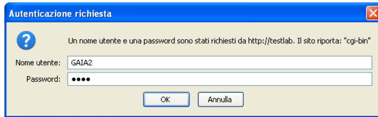
Figura 3. Richiesta autenticazione.
