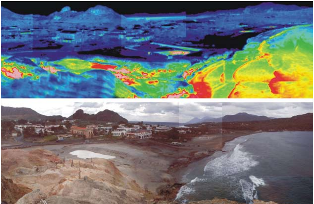
Fig.1 - Immagine all'infrarosso dell'area della Baia di Levante. Le aree calde sono rappresentate dai colori verde, giallo, rosso e rosa (ordine crescente di temperatura). Modificato da CHIODINI et al. (2005).
