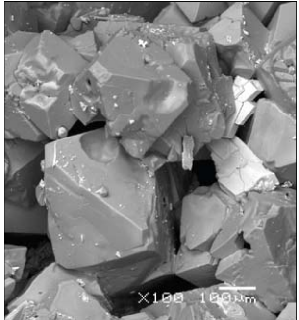
A sinistra. Alum-(K) - Rozzi cristalli ottaedrici sino a 0,5 mm associati a calcantite. Grotta dell'Allume, aprile 2008. A destra. Alum-(K) - Cristalli ottaedrici sino a 0,5 mm. Grotta dell'Allume, aprile 2008.
