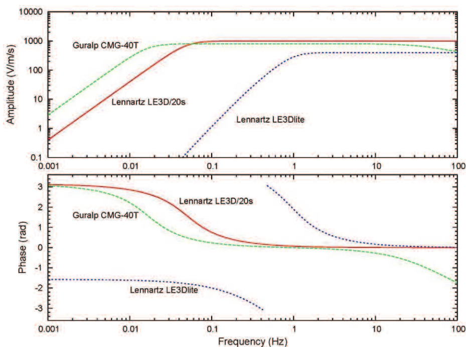
Figure 5 Amplitude (top) and phase (bottom) of the transfer functions for the three sensors used in the Mobile Seismic Network. Figura 5 Ampiezza (sopra) e fase (sotto) della funzione di trasferimento per i tre diversi sensori utilizzati dal Mobile Seismic Network.
