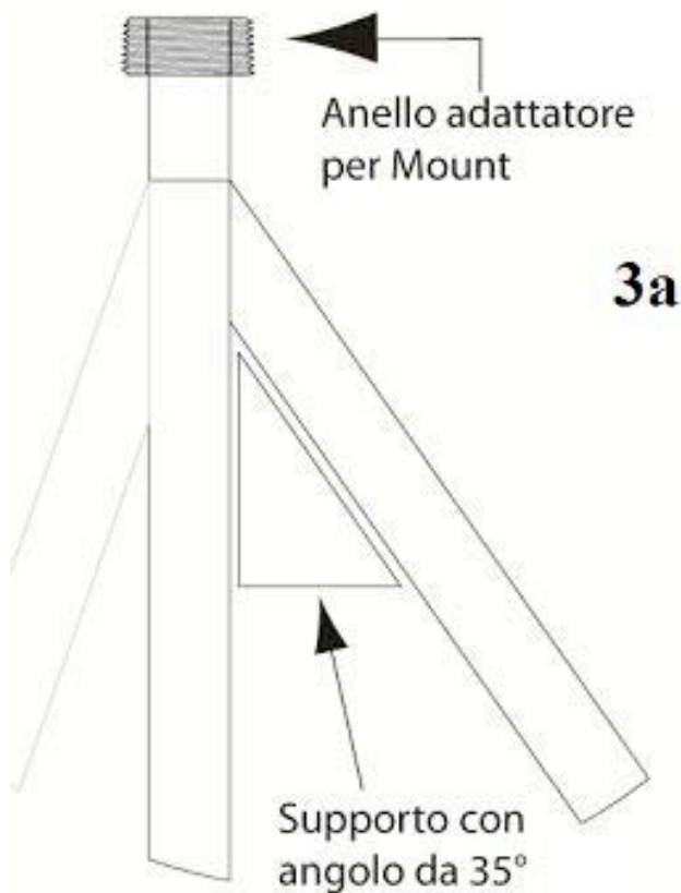
Figura 3. a) Progetto del raccordo tra aste laterali e asta centrale e dell'anello adattatore tronco conico del tripode superficiale tipo "Wyatt/Agnew"; b) Foto dell'anello adattatore tronco conico e dei supporti ad angolo di 35° assemblati.
