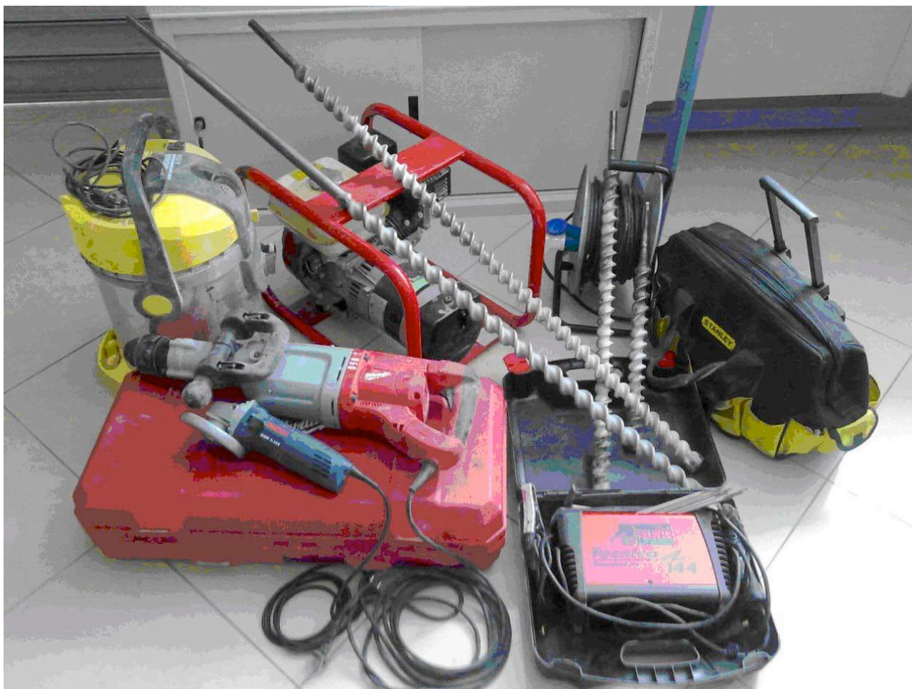
Figura 6. Attrezzature utilizzate per la realizzazione dei monumenti tipo short-drilled-braced .
