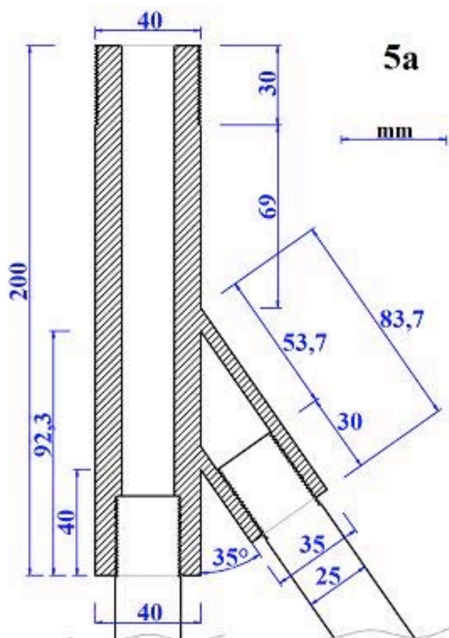
Figura 5. a) Progetto del nuovo tipo di adattatore tripode progettato per migliorare ulteriormente la realizzazione di monumenti tipo short-drilled-braced 4EVO (versione 3); b) Foto del nuovo adattatore tripode.
