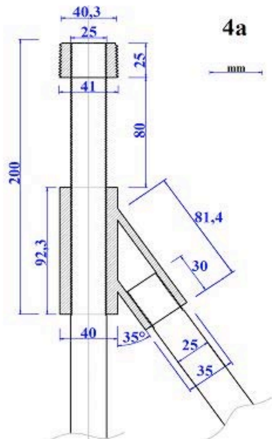
Figura 4. a) Progetto del raccordo tra aste laterali e asta centrale e dell'anello adattatore filettato del tripode superficiale modello D'Ambrosio (versione 2); b) Foto dell'adattatore tripode e dell'anello adattatore assemblati.
