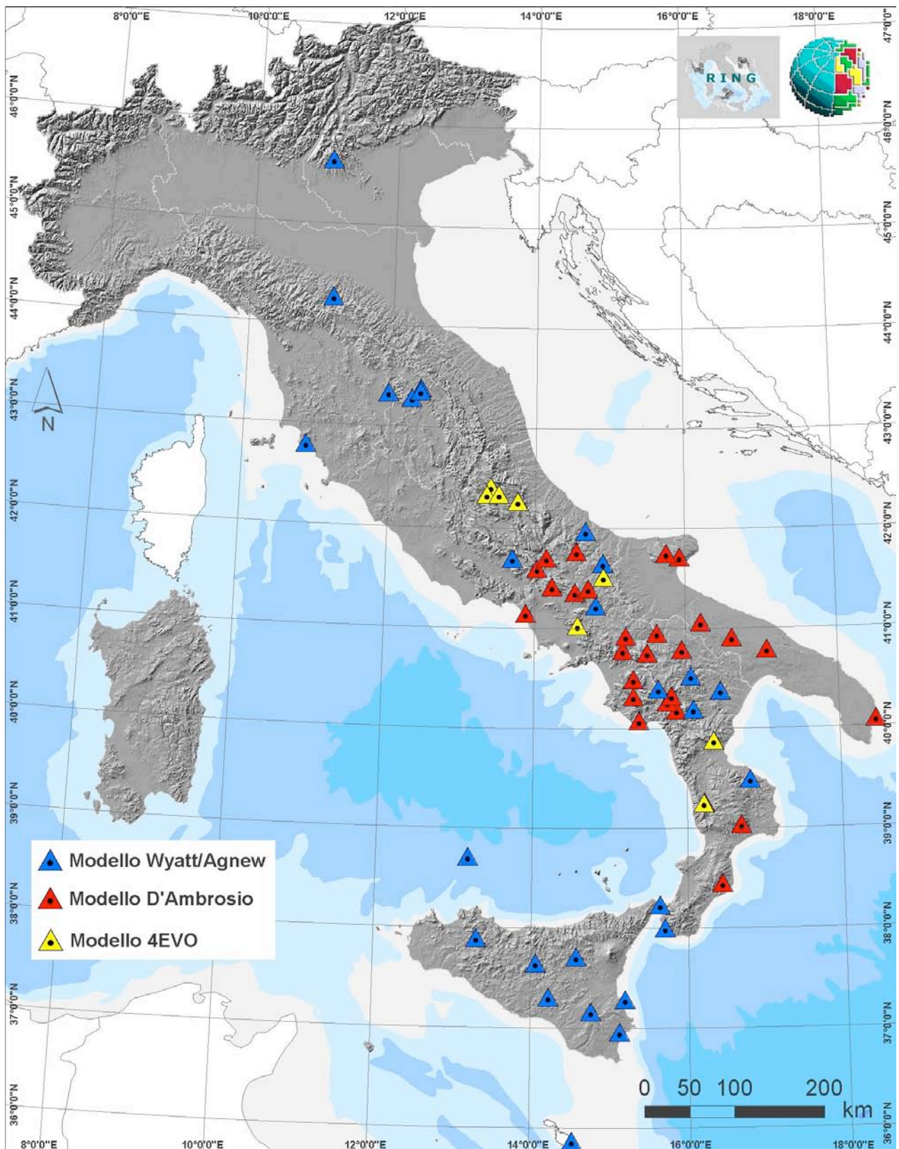
Figura 10. Monumenti realizzati con tripodi superficiali all'interno della RING. I dettagli dei siti sono riportati nell'allegato 2.
