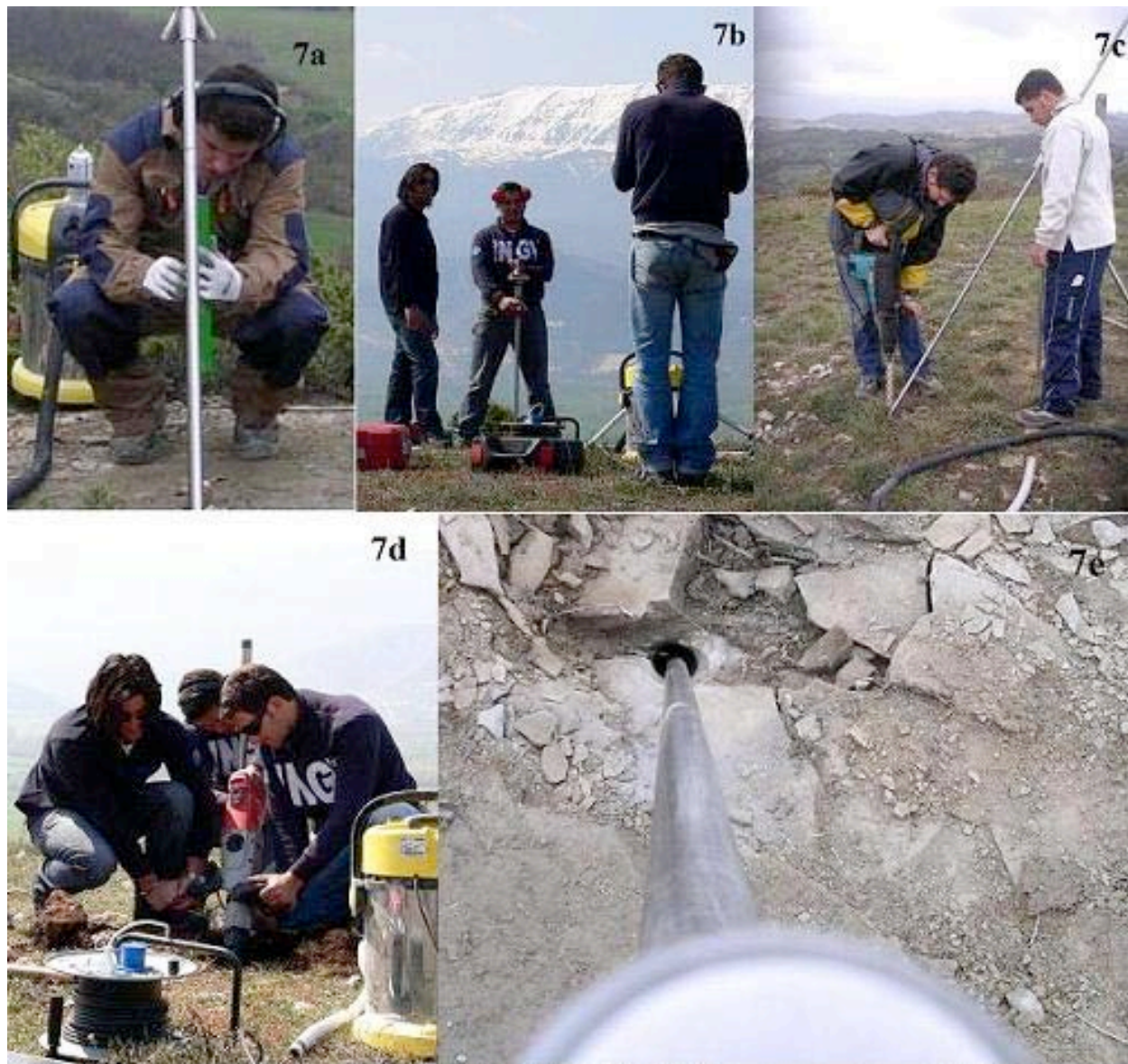
Figura 7 (a, b, c, d, e). Fasi di installazione del monumento GPS permanente tipo short-drilled-braced . Per i dettagli si veda il testo.
