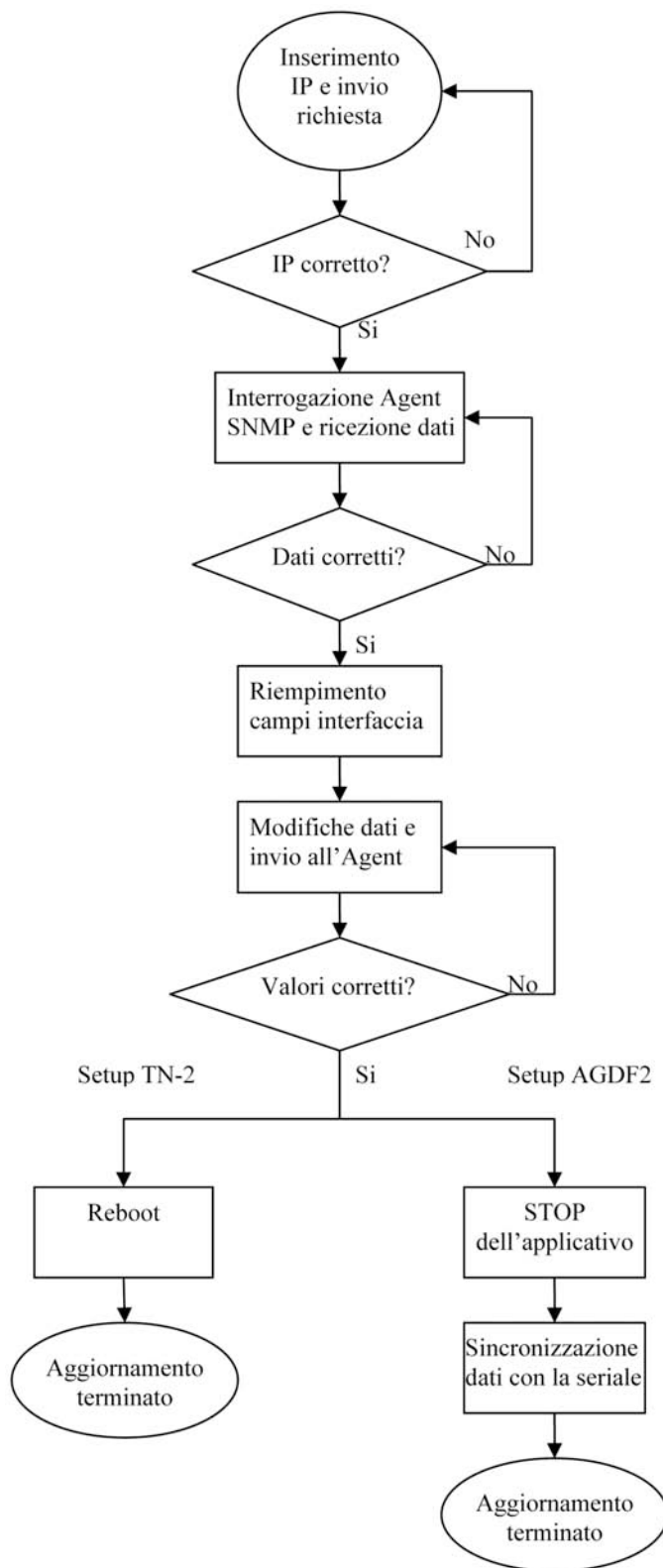
Figura 12. Diagramma di flusso di GAIA setup.
