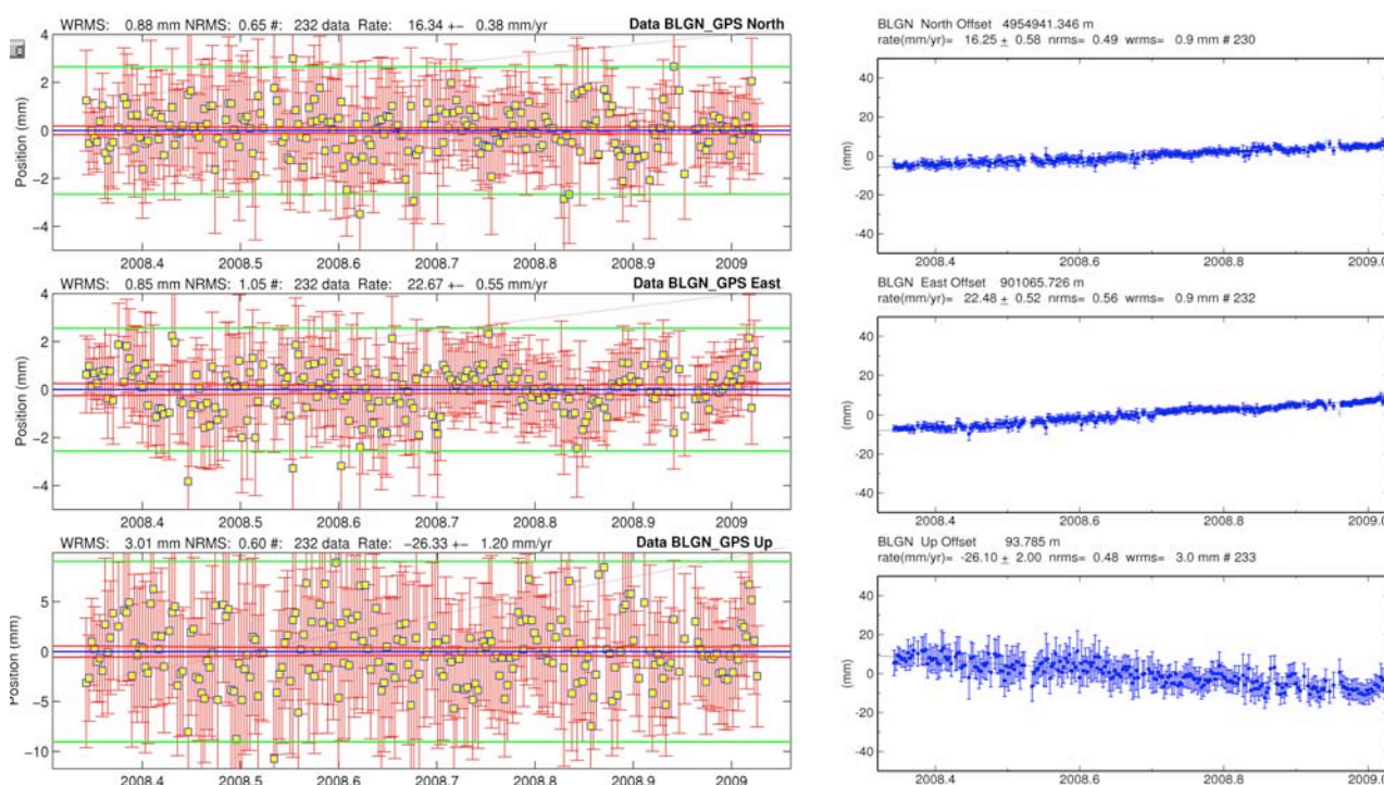
Figura 5. Serie temporali della stazione permanente di BLGN ottenute con l'ausilio dei programmi tsview ed enfit , rispettivamente appartenenti al pacchetto matlab-tools e Globk . Si noti come entro la tolleranza degli errori i valori delle componenti di velocità stimate sono ripetibili.
