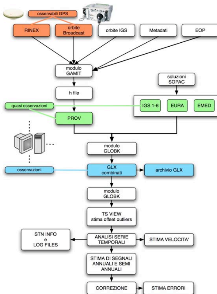
Figura 4. Diagramma di flusso dell'archiviazione e processamento del dato GPS; in marrone, verde e blu vengono evidenziati rispettivamente: gli osservabili GPS, le quasi osservazioni ( h-files ) e le osservazioni.
