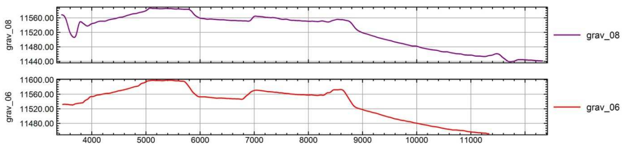
Figura 14: Confronto di due linee ripetute esattamente lungo la cresta sommitale del Vulcano Marsili (2006-2008).
