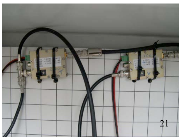
Figura 21. I due trasmettitore video MTX 2100 da 100 mW settati a 2100 Mhz e 1600 Mhz.
