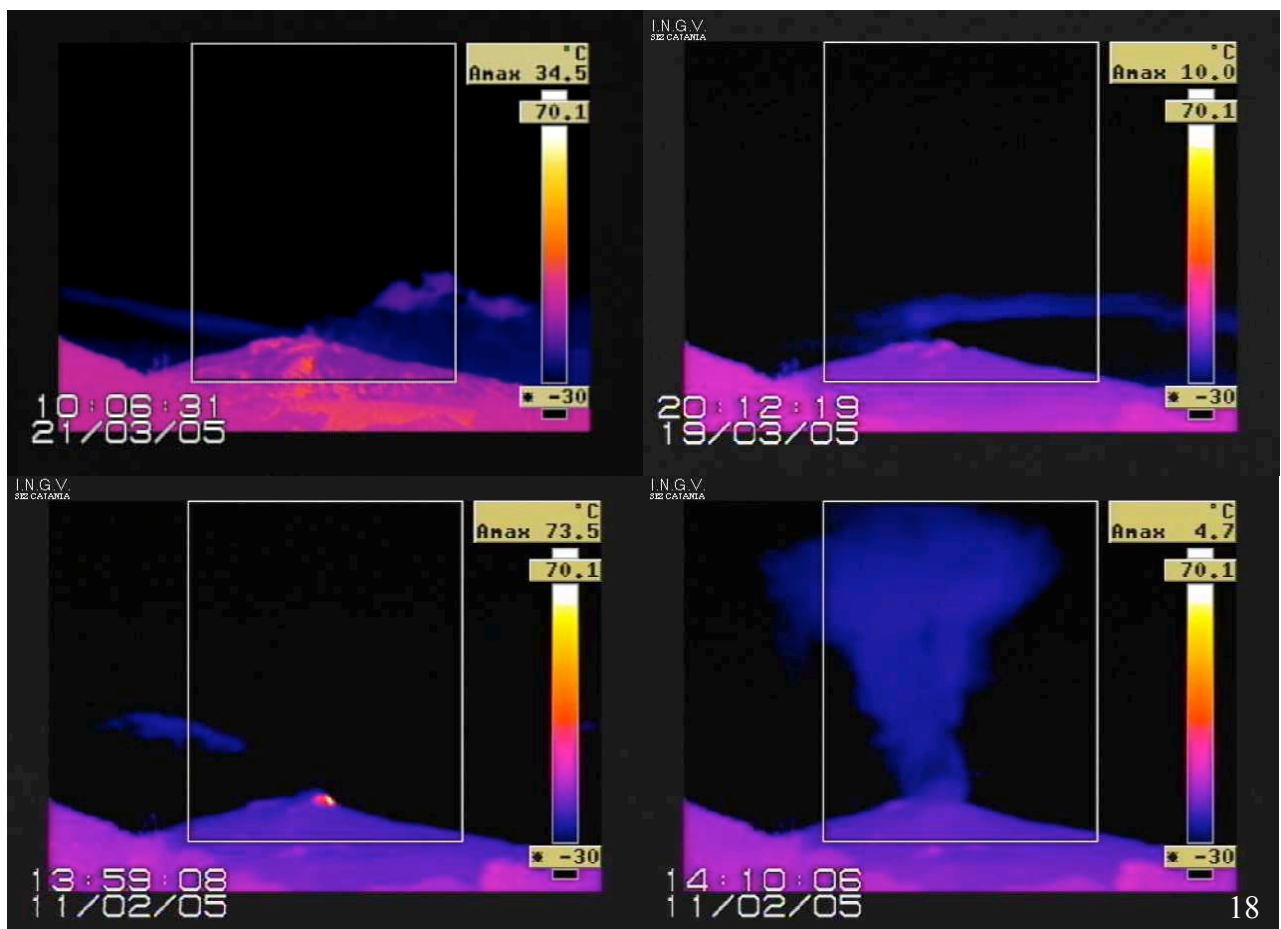
Figura 18. Immagini del 2005 dell'Etna riprese dalla telecamera termica Flir 320 M installata a Nicolosi.
