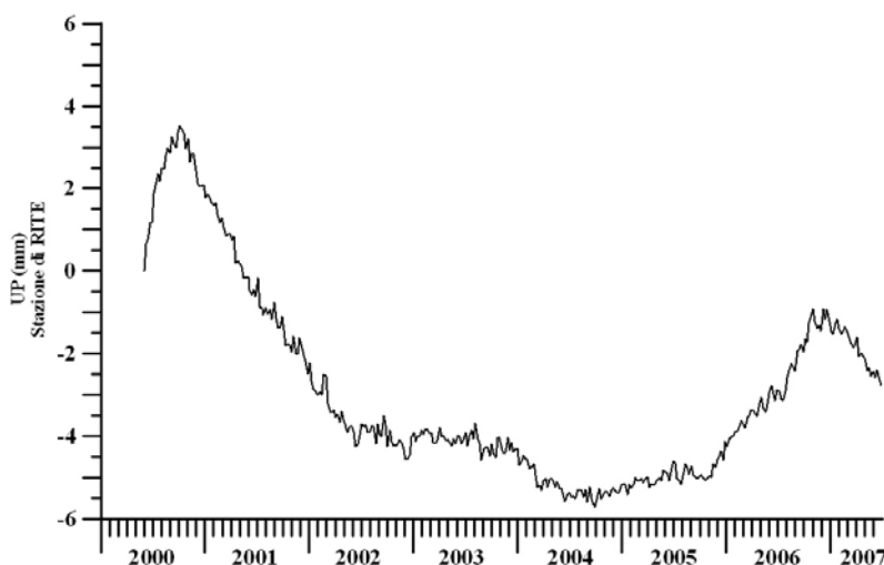
Figura 5 - Serie temporale, da maggio 2000 a giugno 2007, delle variazioni settimanali in Up della stazione GPS di RITE (Rione Terra).
