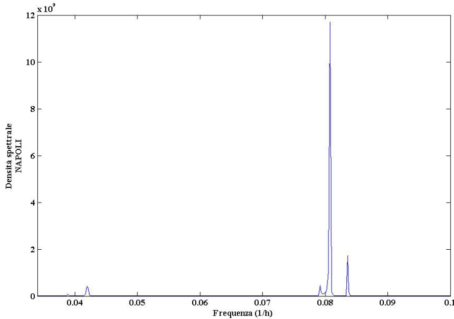
Figura 3 - Spettro del livello del mare misurato a Napoli. Viene mostrato l'intervallo di frequenze caratteristico delle componenti diurne e semidiurne.
