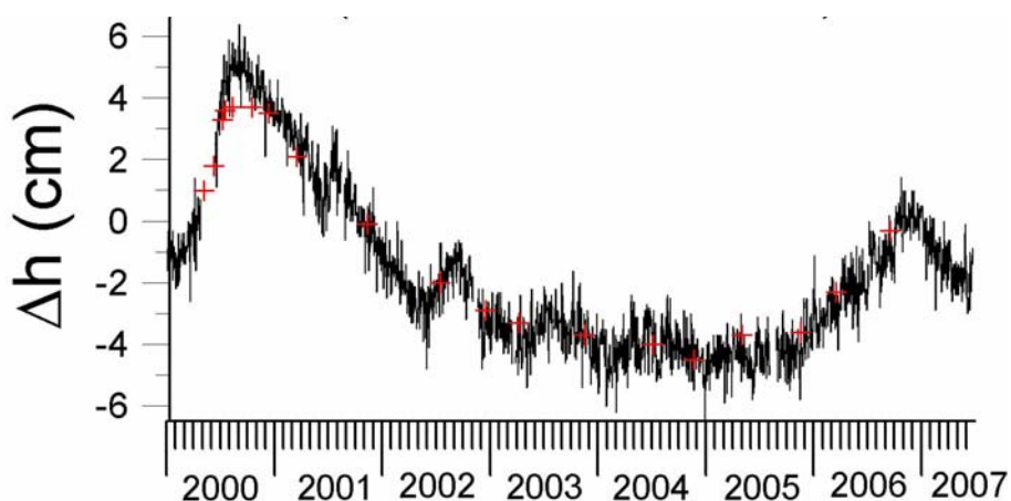
Figura 4 - Deformazione verticale del suolo dedotta da dati mareografici, dal 1/1/2000 al 30/06/2007, per il sito di Pozzuoli, confrontata con quella determinata dalla livellazione geometrica (croci).
