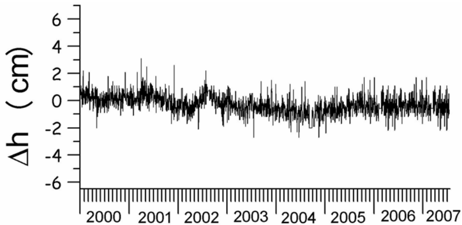
Figura 6 - Deformazione verticale del suolo dedotta da dati mareografici, dal 1/1/2000 al 30/06/2007, per il sito di Torre del Greco.
