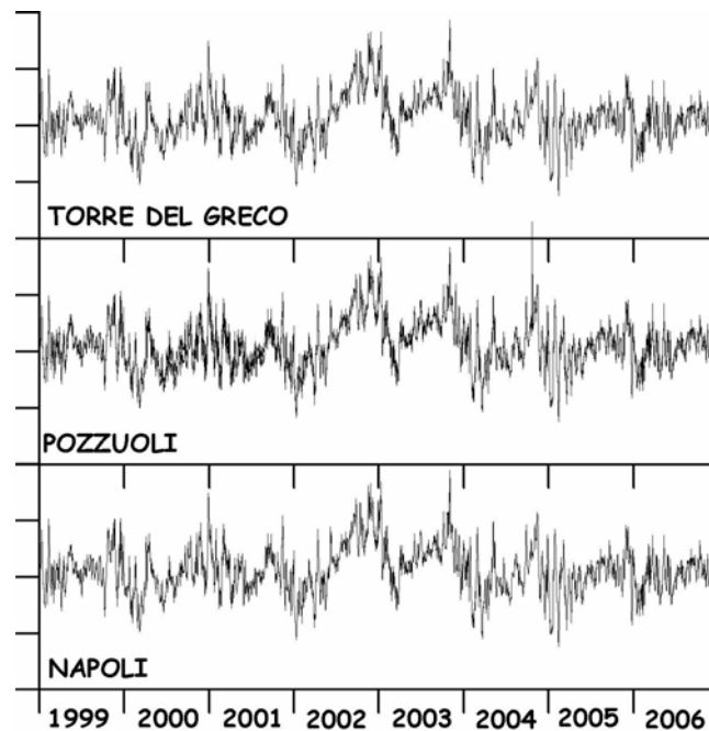
Figura 2 - Esempio di segnale mareografico registrato dai sensori analogici dal gennaio 1999 al dicembre 2006. Sulla scala verticale ogni tacca corrisponde a 20 cm.
