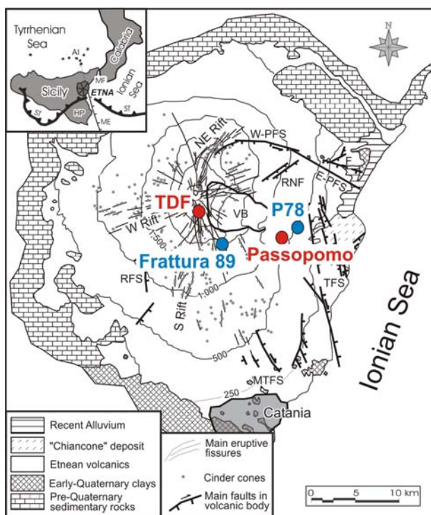
Fig. 5 – Ubicazione dei siti di misura delle concentrazioni di Hg e del flusso di CO 2 nei suoli. Nei siti TDF e P78 le misure sono state ripetute nel tempo. Mappa strutturale modificata da Neri et al (2004).
