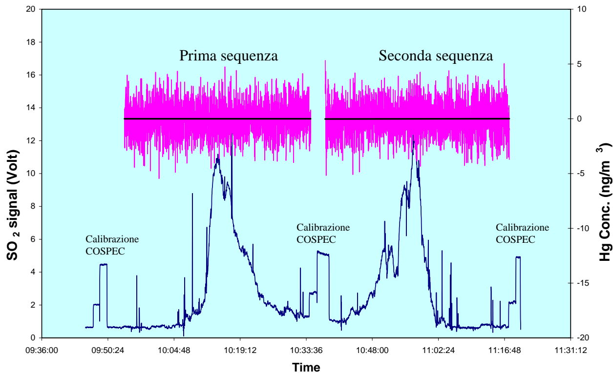
Fig. 2 - Misure combinate in continuo del segnale di SO_2 ottenuto dal COSPEC (linea blu, ordinate di sinistra) e della concentrazione di Hg (linea viola, ordinate di destra) effettuate il giorno 7 Dicembre 2005 lungo la strada da Zafferana Etnea verso Linguaglossa (prima sequenza) e ritorno (seconda sequenza). I valori (gradini) di concentrazione di riferimento delle calibrazioni dello strumento COSPEC sono di 128 ppm•m (parti per milione per metro, gradino o valore più basso) e 406 ppm•m (gradino o valore più elevato).
