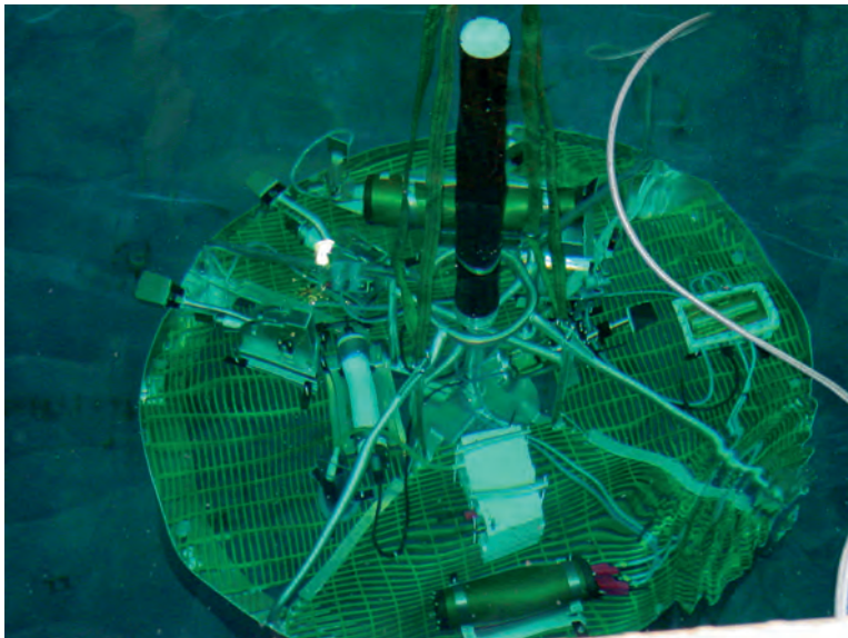
Fig. 6. ASSEM node.
