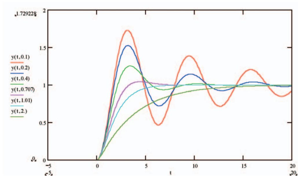
Figura 3 Andamento delle oscillazioni di un sistema del secondo ordine (con pulsazione di risonanza unitaria) forzato con un gradino unitario, e parametrizzato con il coefficiente di smorzamento \xi .
