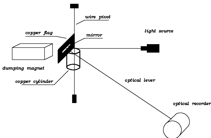
Figura 11. Il sismografo Wood-Anderson .
