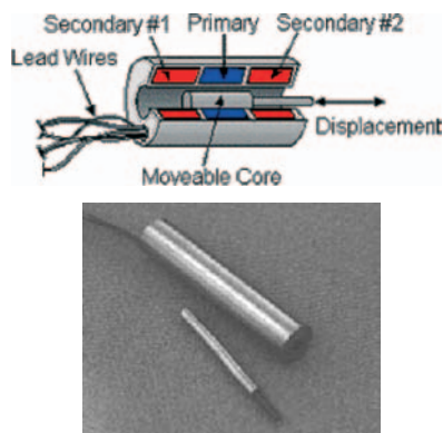
Figura 13 Rivelatore di posizione LVDT. A sinistra è mostrato uno spaccato del dispositivo, mentre a destra si vede l'aspetto di un componente commerciale. Il cilindro di dimensioni maggiori è il trasformatore privo del nucleo mobile, quello più piccolo è il nucleo.
