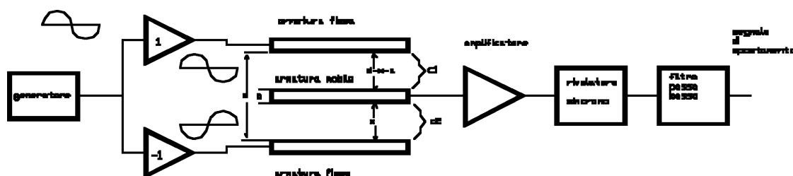
Figura 12 Rivelatore di posizione capacitivo. Le due armature fisse sono polarizzate con tensione alternata in opposizione di fase. La tensione rivelata sull'armatura mobile è proporzionale alla posizione assunta da quest'ultima (vedi testo).
