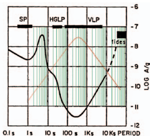
Figura 28 La risposta in accelerazione di un sismografo a larga banda confrontato con lo spettro in accelerazione del rumore sismico.
