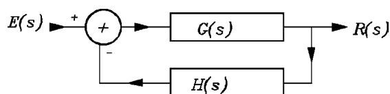
Figura 20 Tipico schema a blocchi di un sistema reazionato; G(s) è detto ramo diretto, mentre H(s) è detto ramo di reazione.
