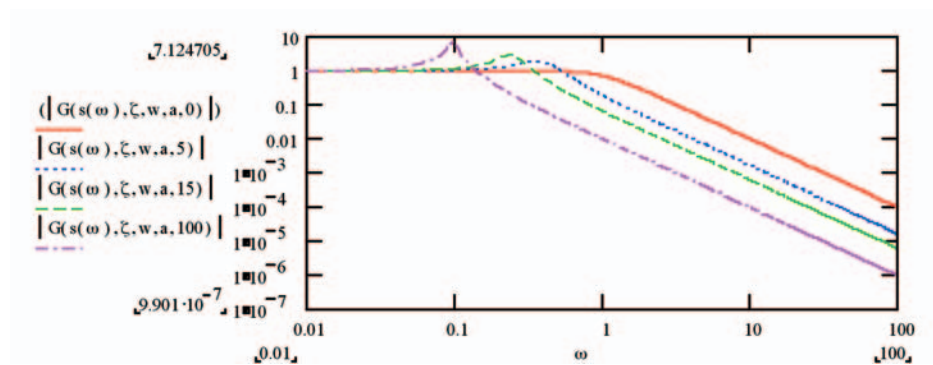
Figura 24 Risposta all'accelerazione di un sismografo con reazione negativa sull'accelerazione.
