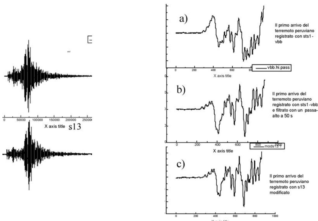
Figura A6_3 Il terremoto peruviano del 7 luglio 2001 visto dall'S13 a banda allargata e da un sts1-vbb.
