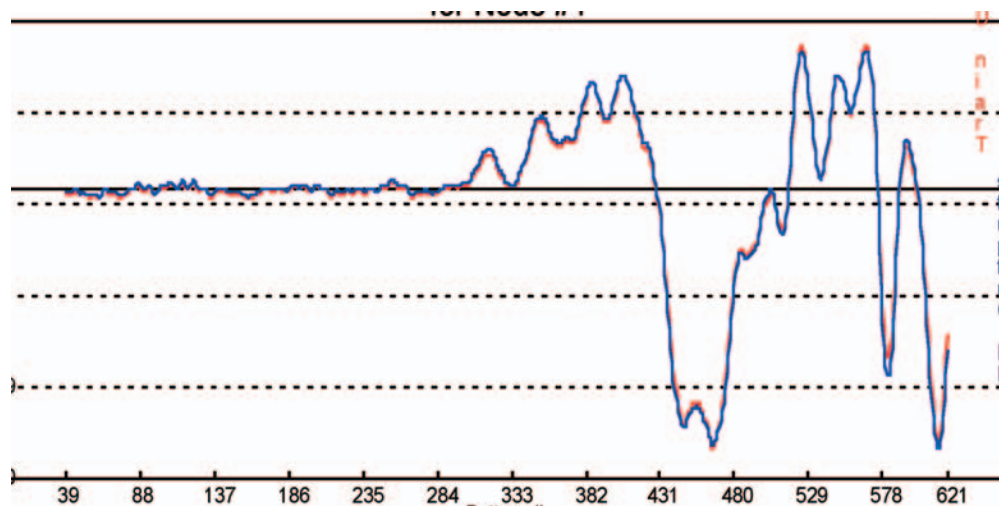
Figura A6_5 Paragone tra s13 allargato e filtrato (traccia rossa) ed il segnale dell' sts1 (traccia blu).
