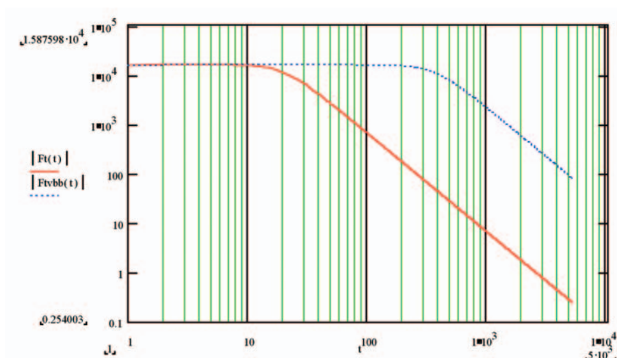
Figura 27 Diagramma della risposta in frequenza dei sismografi STS-1 (rosso) ed STS-1 VBB (blu).
