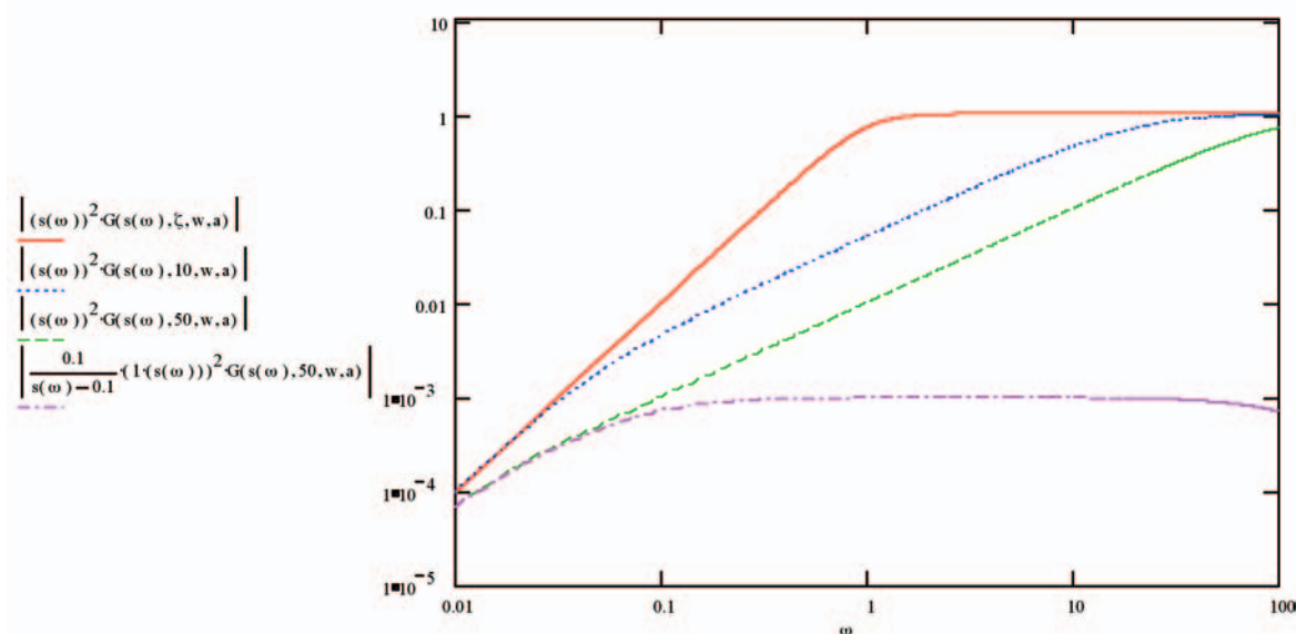
Figura 18 La curva in rosso rappresenta la risposta in frequenza di un geofono ( \xi=1/\div 2 ) eccitato con un segnale di velocità. Le curve in blu e verde mostrano come la curva di risposta si modifichi ponendo rispettivamente \xi=10 e \xi=50 . La curva in viola rappresenta la risposta filtrata attraverso un passa-basso con un polo per \omega=0.1 \text{ s}^{-1} . Dopo questo trattamento la risposta dello strumento diviene piatta sulle velocità in un cospicuo intervallo di frequenza (quasi 3 decadi).
