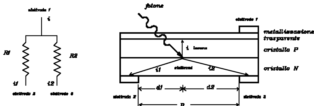
Figura 15 Rivelatore di posizione ottico analogico PSD. La posizione del punto luminoso sulla superficie del sensore è funzione dei rapporti delle correnti sugli elettrodi (vedi testo).
