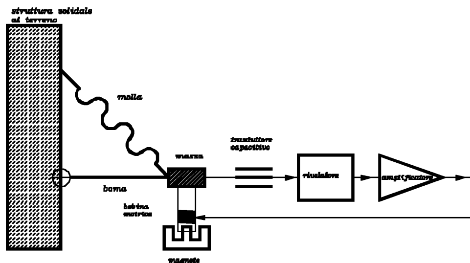
Figura 19 Sismografo a reazione negativa. Il segnale di posizione della massa ottenuto attraverso un trasduttore capacitivo, viene inviato alla bobina motrice che esercita una forza sulla massa stessa.
