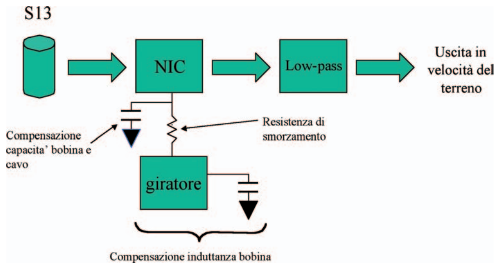
Figura A6_1 Schema a blocchi dell'estensore di banda di tipo Lippman applicato all'S13.
