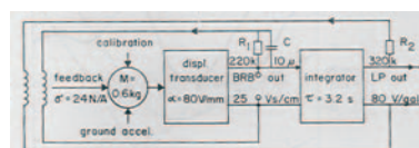
Figura 25 Schema di principio del sismografo STS-1.
