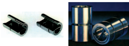
Figura 8 Pivots ad attrito nullo. La sospensione si basa sulla flessione di due lame d'acciaio. Per piccoli angoli la coppia di ritorno è lineare con l'angolo e la vita del dispositivo è indipendente dal numero dei cicli.
