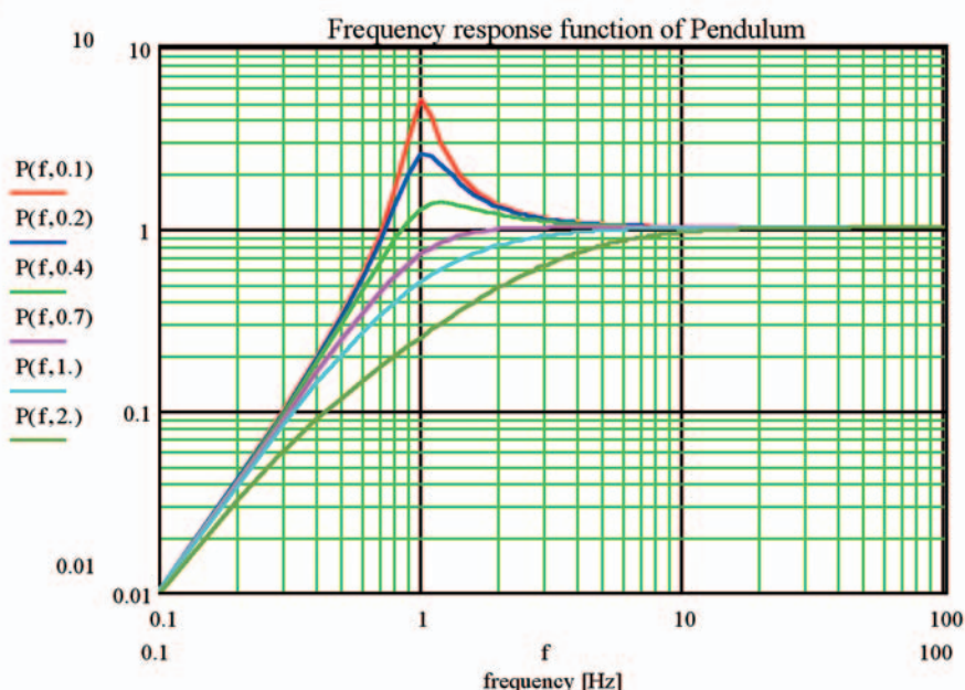
Figura 4 Diagramma della risposta di un pendolo allo spostamento del terreno.
