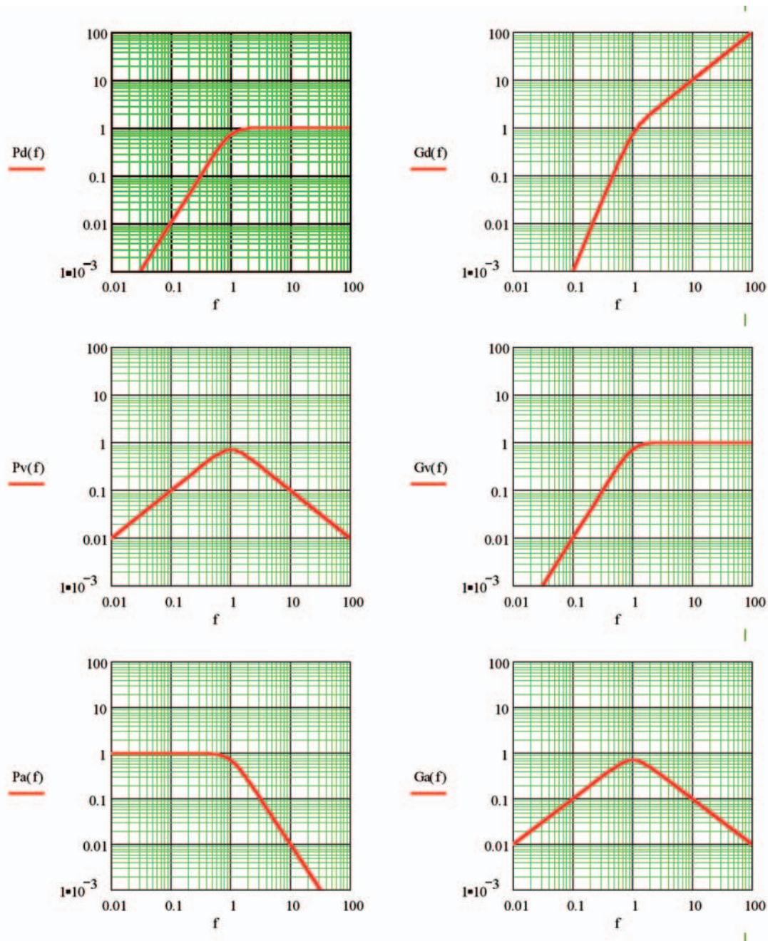
Figura 5 Andamento delle funzioni di trasferimento di un pendolo (colonna di diagrammi a sinistra) e di un geofono (colonna di diagrammi a destra) eccitati con segnali di spostamento (prima linea di diagrammi); di velocità (seconda linea di diagrammi) e di accelerazione (terza linea di diagrammi).
