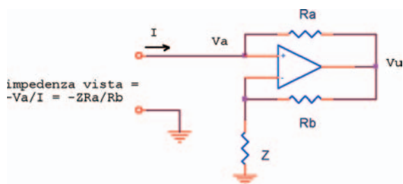
Figura A5 Schema di un circuito NIC ( Negative Impedance Converter ).
