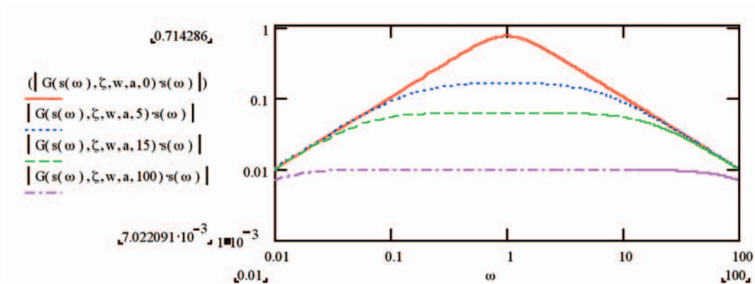
Figura 23 Risposta alla velocità di un sismografo con reazione negativa sulla velocità.
