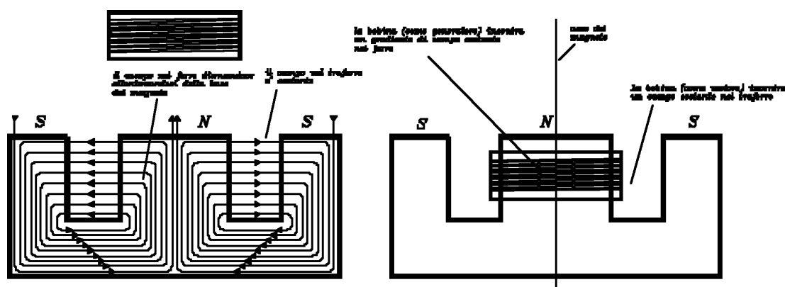
Figura 16 Rivelatore elettromagnetico di velocità. Il magnete è costruito in modo da avere flusso costante nel ferro (e gradiente costante nel traferro). La figura a sinistra mostra, in alto la bobina e, in basso il magnete, dove sono evidenziate le linee di forza. A destra la bobina è posta nella sua posizione di lavoro. La fem ai capi della bobina è proporzionale alla velocità con cui la bobina si muove nella direzione dell'asse del magnete.
