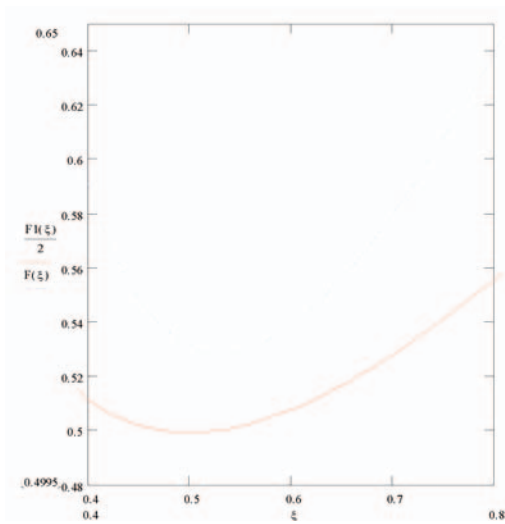
Figura A2 Diagramma delle funzioni di errore (minimo quadrato) della funzione di trasferimento e della risposta all'impulso in funzione del coefficiente di smorzamento.
