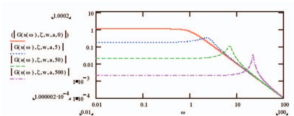
Figura 21 Risposta di un sistema con reazione di posizione parametrizzato con il coefficiente di guadagno di reazione.
