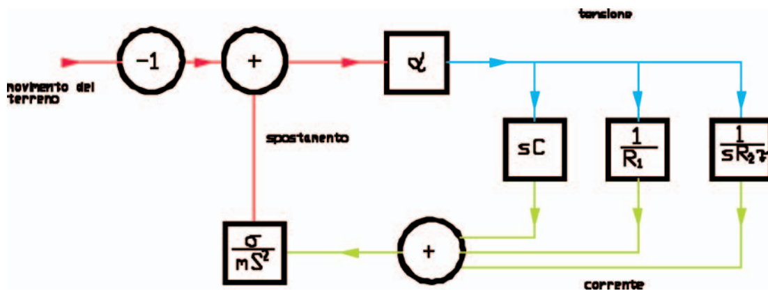
Figura 26 Schema di principio del sismografo STS-1 disegnato con blocchi funzionali. Le grandezze fisiche che vengono trasferite dai vari blocchi appaiono in colori diversi: in rosso gli spostamenti, in blu le tensioni ed in verde le correnti.
