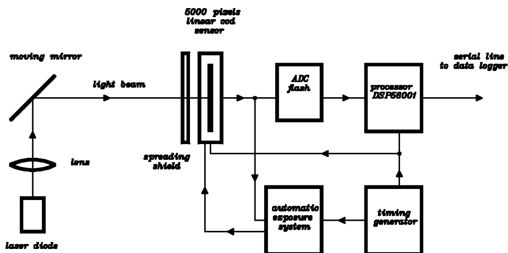
Figura 14 Schema a blocchi del rivelatore di posizione ottico basato su una CCD. Un microcalcolatore (DSP) calcola il centro della distribuzione della luce sull'elemento sensibile, e fornisce in uscita un risultato numerico.
