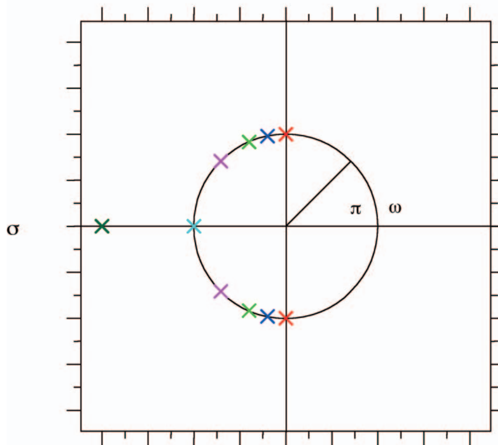
Figura A8 Diagramma Poli-Zeri per un sismometro a 1 \text{ Hz} con diversi valori di smorzamento.
