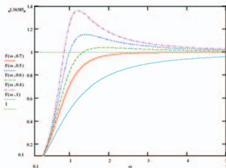
Figura A3 La rappresentazione in scala bilineare della funzione di trasferimento evidenzia la presenza dei massimi ed il loro spostamento verso le alte frequenze all'aumentare del coefficiente di smorzamento.
