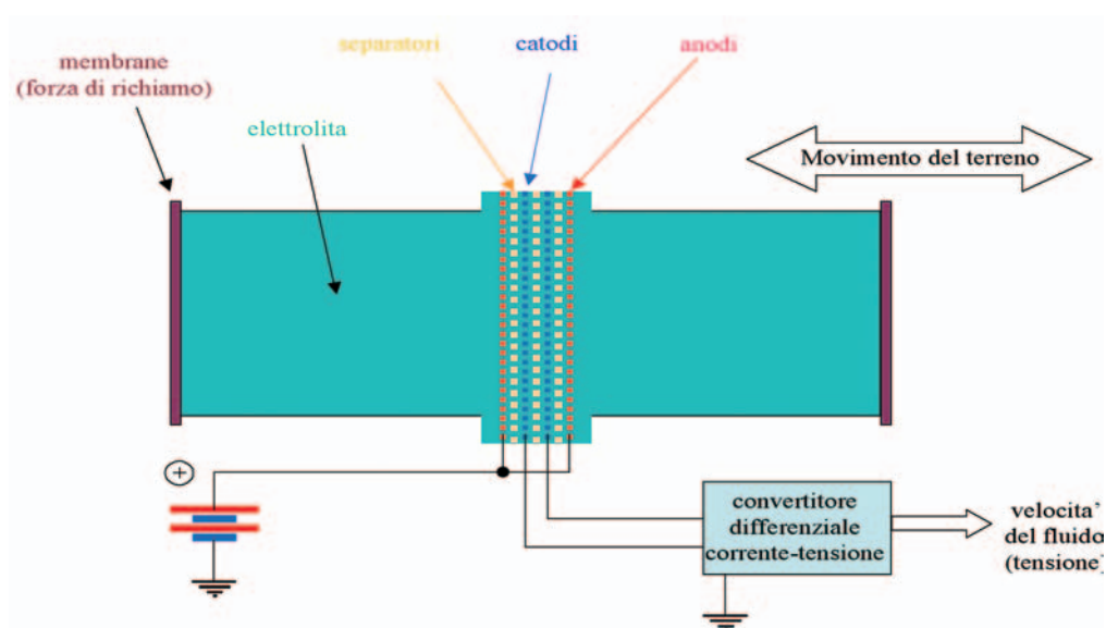
Figura 29 Esempio di trasduttore MET applicato ad un sismografo. Il recipiente visualizzato in una sezione passante per l'asse di sensibilità è riempito con un elettrolita e trattenuto alle estremità da due membrane elastiche. La velocità del moto del liquido è rivelata dall'insieme di elettrodi che costituisce il trasduttore MET (vedi testo).
