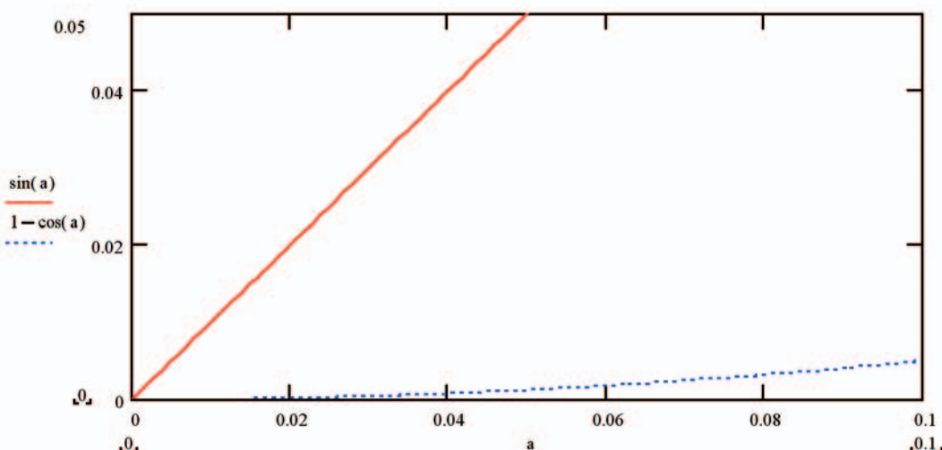
Figura 10 Andamento delle accelerazioni su un sismografo verticale (linea tratteggiata) e su un sismografo orizzontale (linea continua) per piccole variazioni dalla verticale.
