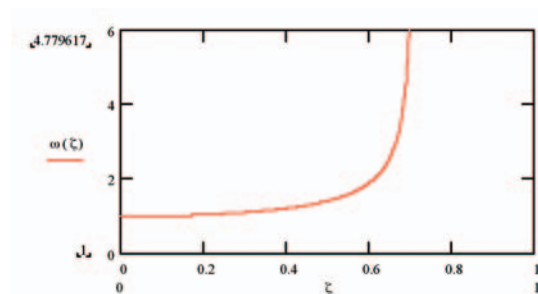
Figura A4 La posizione dei massimi (ordinate) in funzione del coefficiente di smorzamento (ascisse). La funzione ha un asintoto verticale per \xi=1/\sqrt{2} .
