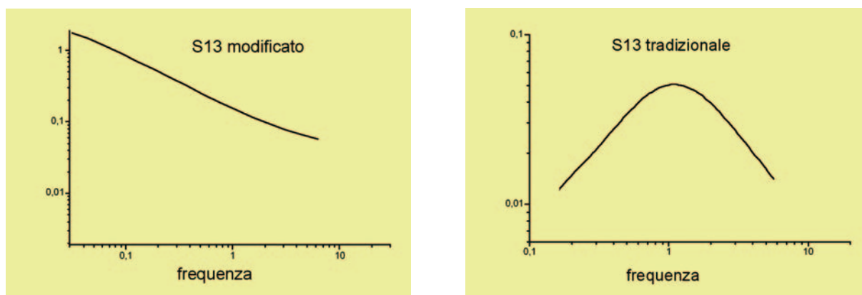
Figura A6_2 Risposta di un s13 tradizionale ed a banda allargata (taglio a 50 s) ad una eccitazione in accelerazione.
