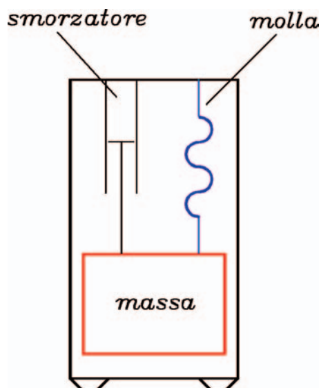
Figura 2 Schema semplificato di un sismografo. La massa è libera di muoversi verticalmente sospesa alla molla; lo smorzatore fa estinguere le oscillazioni indotte nel sistema massa-molla.
