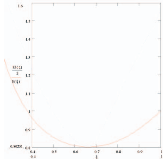
Figura A1 diagramma delle funzioni di errore (minimo modulo) della funzione di trasferimento e della risposta all'impulso in funzione del coefficiente di smorzamento.
