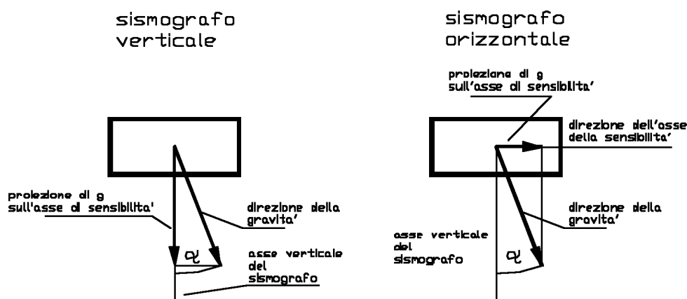
Figura 9 Effetto della variazione dell'inclinazione su un sismografo orizzontale ed un sismografo verticale.
