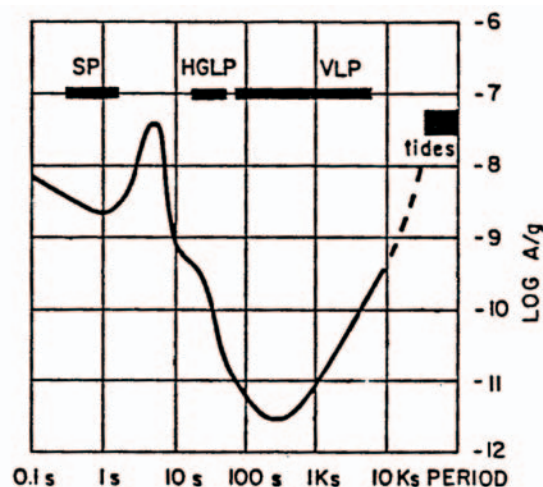
Figura 1 Andamento schematico del rumore sismico.
