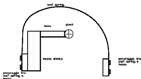
Figura 7 Sagoma di una sospensione leaf-spring . La molla è costruita con una unica lama elastica, naturalmente dritta, che i vincoli costringono ad assumere la sagoma rappresentata nella figura. Come la sospensione Lacoste può essere regolata perché il sistema abbia equilibrio indifferente.
