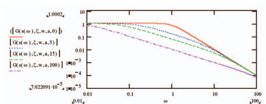
Figura 22 Risposta di un sistema con reazione di velocità parametrizzato con il coefficiente di guadagno di reazione.
