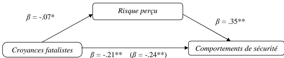
Figure 15 : Médiation partielle de l'effet des croyances fatalistes sur les comportements de sécurité par le risque perçu.
