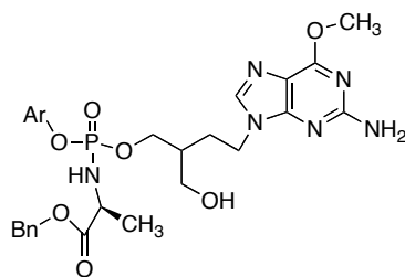
6.4a Ar: Ph 6.4b Ar: 1-NaPh
