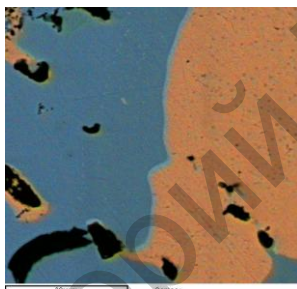
Рис. 1 Плоскость шлифа композиционного материала, полученного с помощью индукционного нагрева
