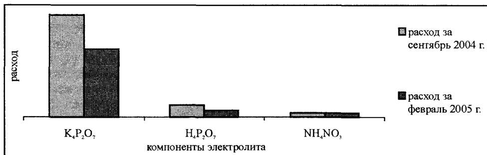
Рис. 2. Расход компонентов электролита щелочного меднения
