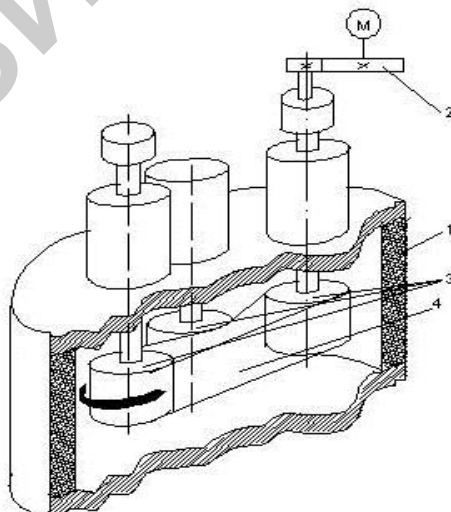
Рисунок 2 – Схема стенда для выбора защитных покрытий для прокатных валков печей отжига листопркатных станков:
