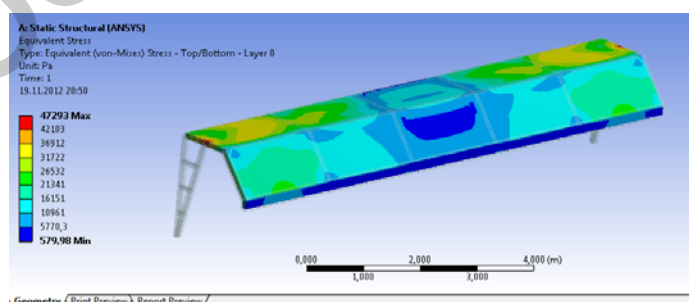
Рисунок 2. Максимальные напряжения, возникающие в укрывающей конструкции при постоянной нагрузке.
