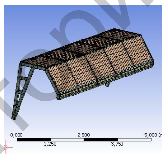
Рисунок 1. Конечно-элементная модель укрывающей конструкции.
