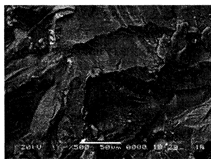
Рис. 3. Усталостный излом сплава, полученного без обработки рафинирующе-модифицирующим комплексом при частоте испытаний 0,3 кГц. ×500
