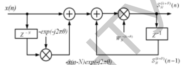
Рисунок 4 – Структура обобщенного КИХ-фильтра, реализующая однобиновое скользящее СДПФ-П на (k + \theta) -ой частоте, при 0 \leq \theta \leq 1 ,
