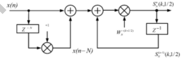
Рисунок 5 – Структура модифицированного КИХ-фильтра, реализующая СДПФ-П на k -й частоте, при \theta = 1/2 .
