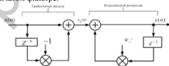
Рисунок 2 – Одна секция комплексного ФОЧВ
