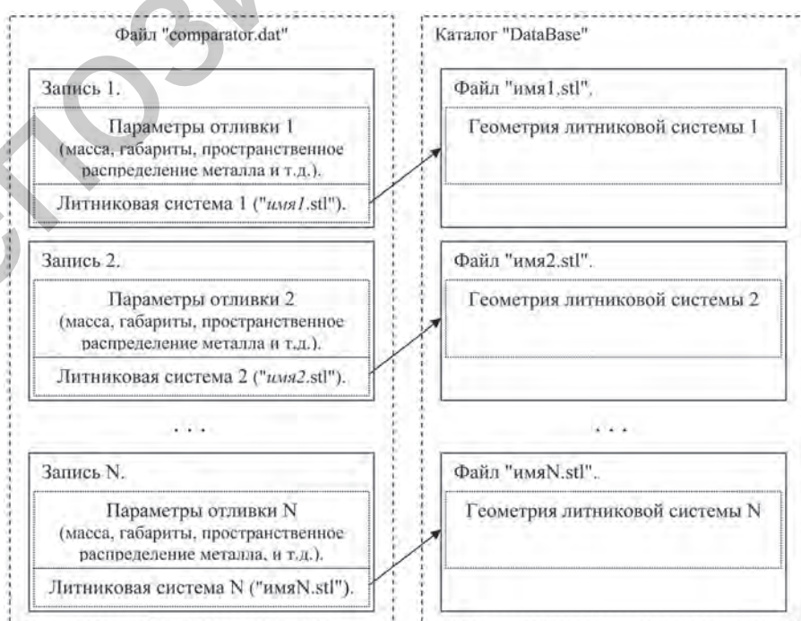
Рис. 1. Структура базы данных для хранения типовых решений «отливка (прототип) – литниковая система»
