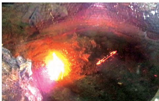
Рис. 5. Состояние рабочей футеровки опытной подины № 4 при стойкости 435 плавков
