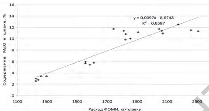
Рис. 3. Зависимость содержания MgO в шлаке от количества присаженного ФОМИ
