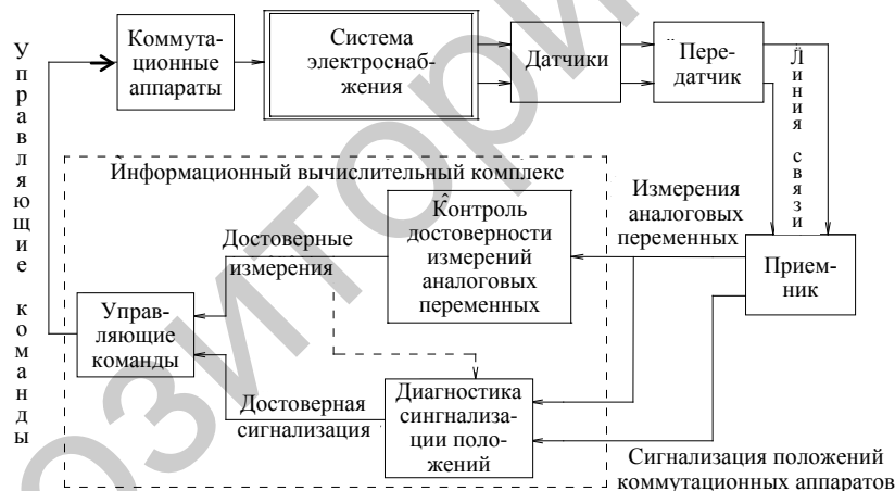
Рис. 1. Схема основных информационных потоков в системе измерений, сбора и обработки измерительной информации
