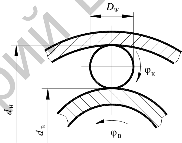
Рисунок 3 – Позиционирование ротора вращением шариков
